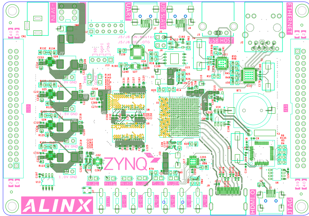
TOP走线层
