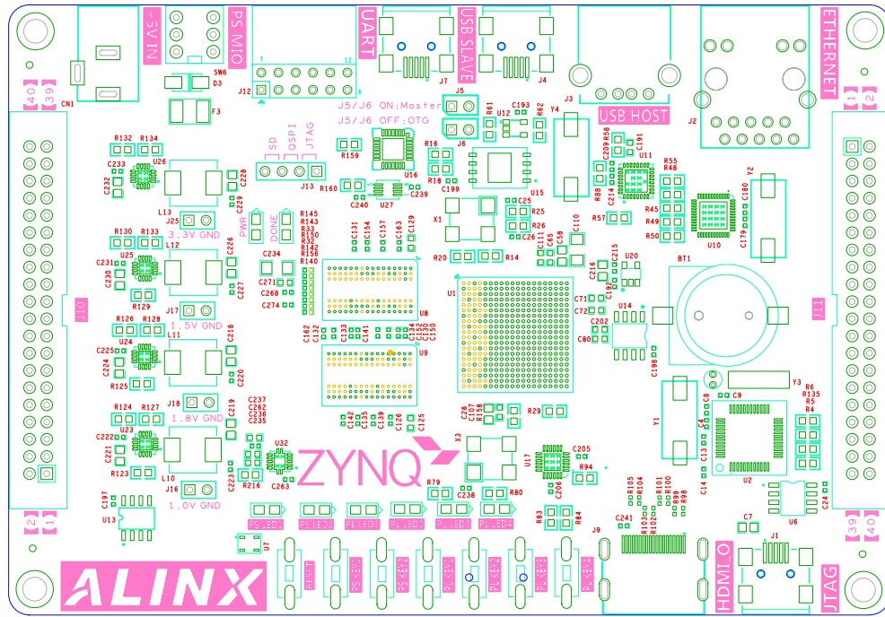
TOP器件层
