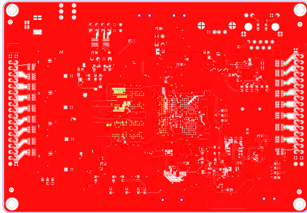
BOTTOM : 走线层
