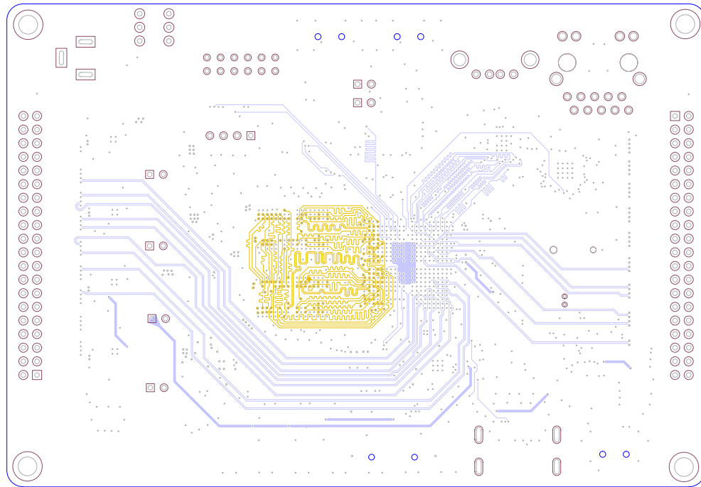
第六层：信号层
