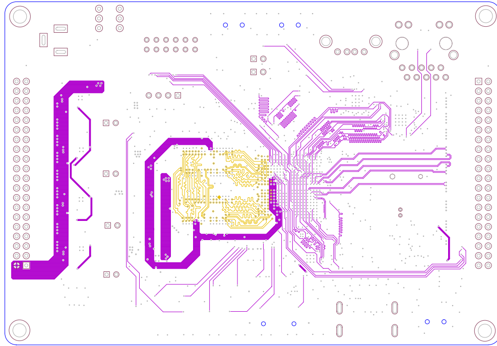
第三层：信号层
