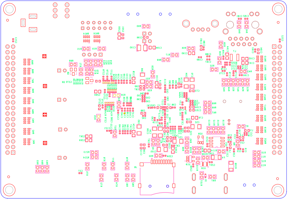
BOTTOM器件层
