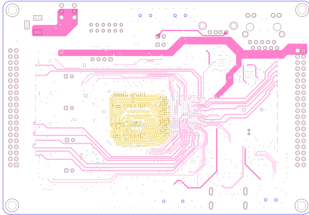
第四层：信号层
